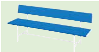
■ベンチBB150 16-40-010 本体¥36,200(税込¥39,820) 19kg H70×D50×W150cm 座/樹脂成形品 脚/スチール □26 粉体塗装
