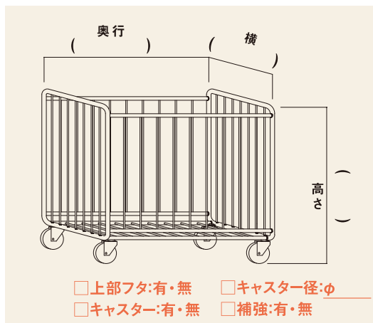
■ボールラック40 (バスケットボール40個収納) 7-17-230 本体¥77,000(税込¥84,700) 高さ182×206×50cm φ27.2 キャスターφ100
